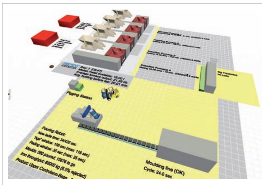
Bild 1: Schmelzbetrieb
